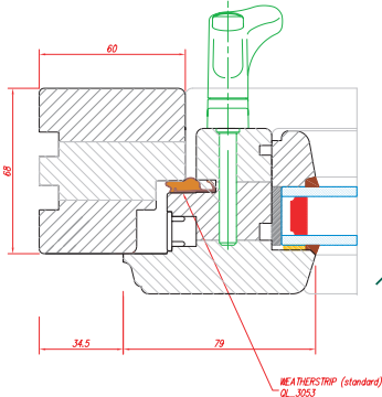
Jamb Section
